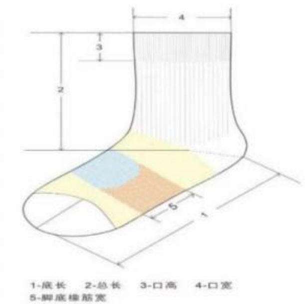
图1 警袜样式及尺寸规格测量方法
