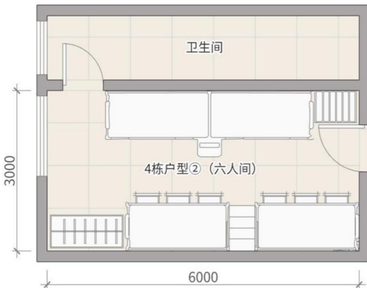
平面布置图
