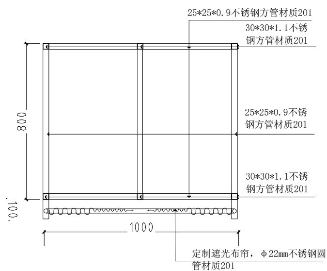
不锈钢柜体平面图
