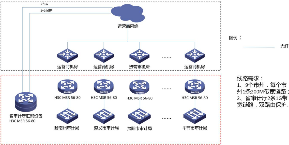
组网拓扑图
