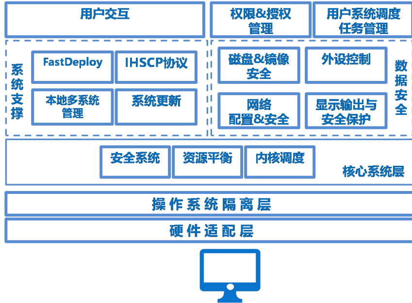
管理运维平台架构图
