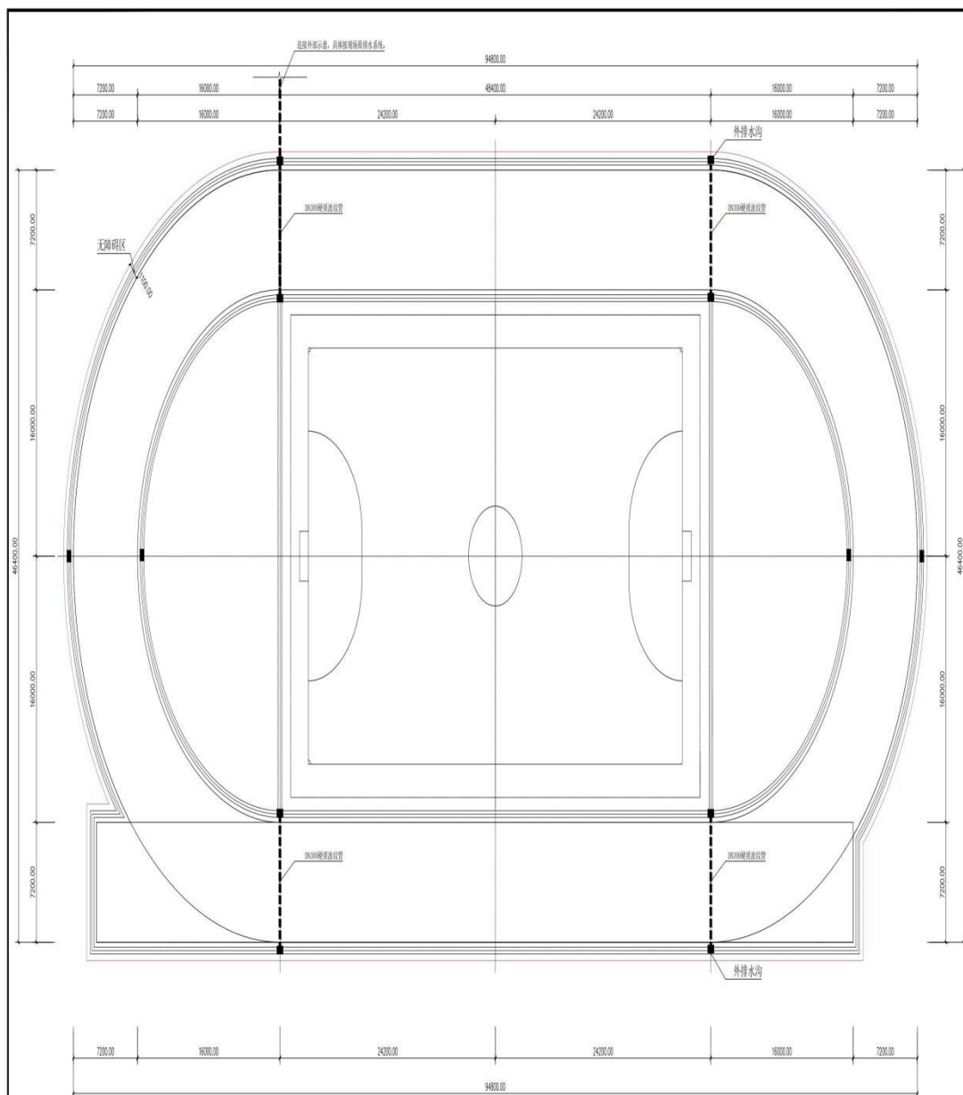
场地排水系统布置图 1:150
