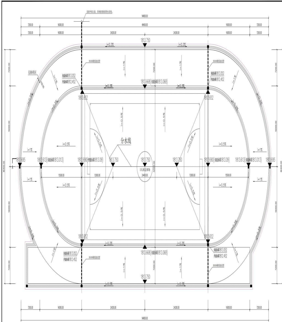
运动场排水、竖向设计平面图 1:150
