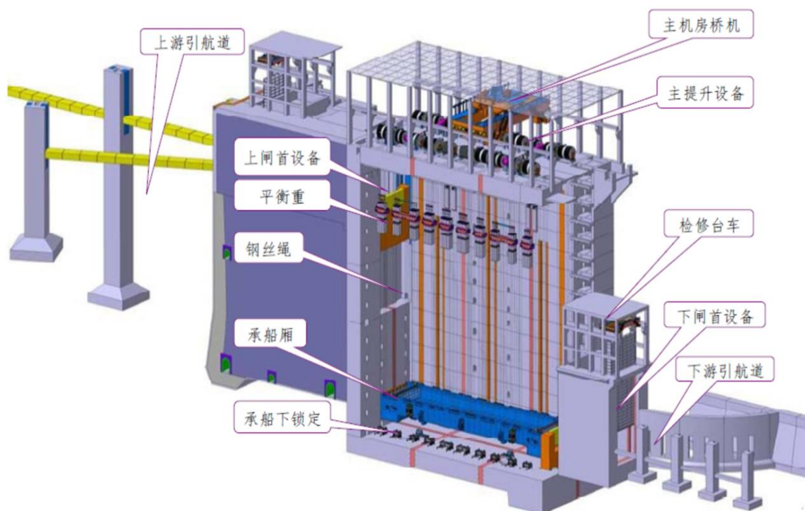
图 1-1 思林升船机总体布置
