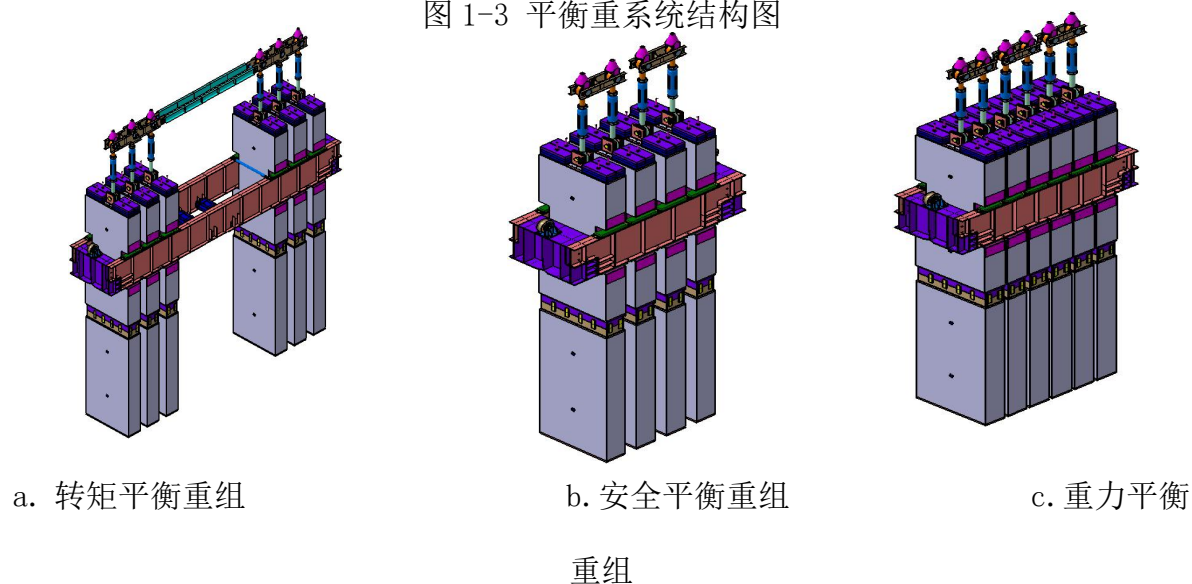
图 1-3 平衡重系统结构图
