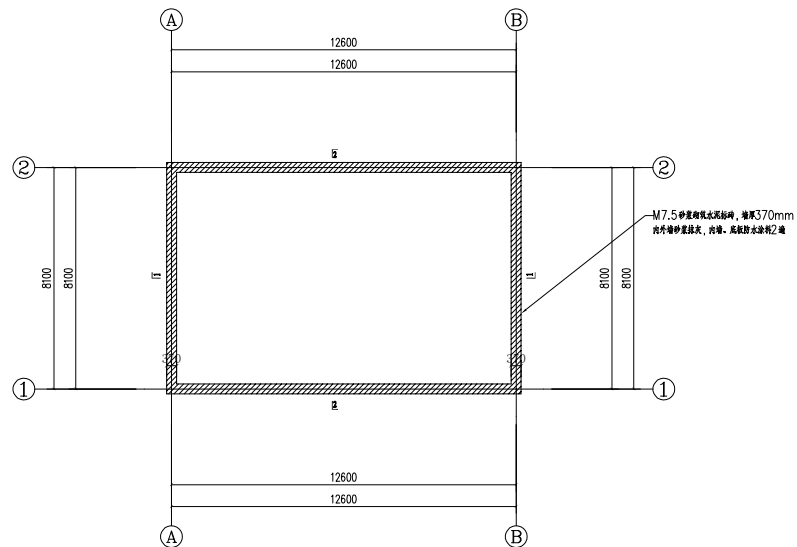
人禽饮水池平面图 1:100
