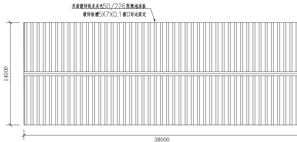
鹅棚(三)屋面平面图 1:100
