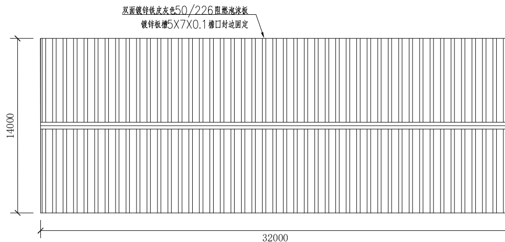
干湿分离区屋面平面图 1:100
