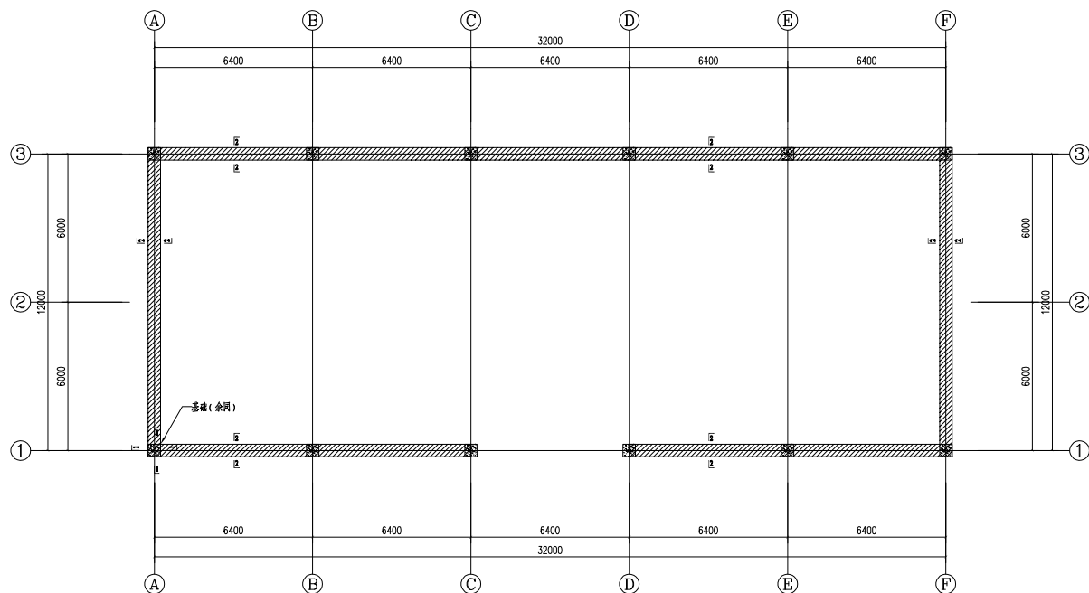
鹅棚(一)基础平面布置图 1:100
