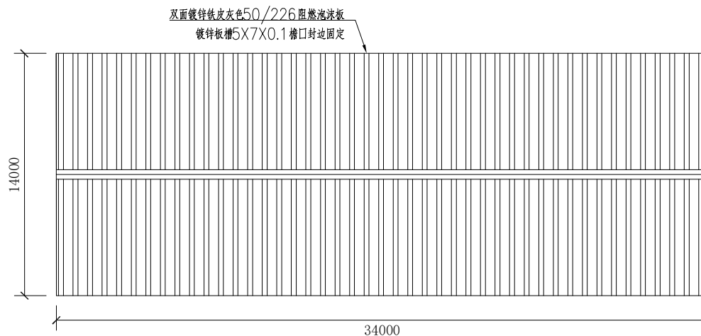
鹅棚(一)屋面平面图 1:100
