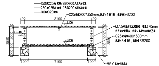
2-2剖面图 1:100
