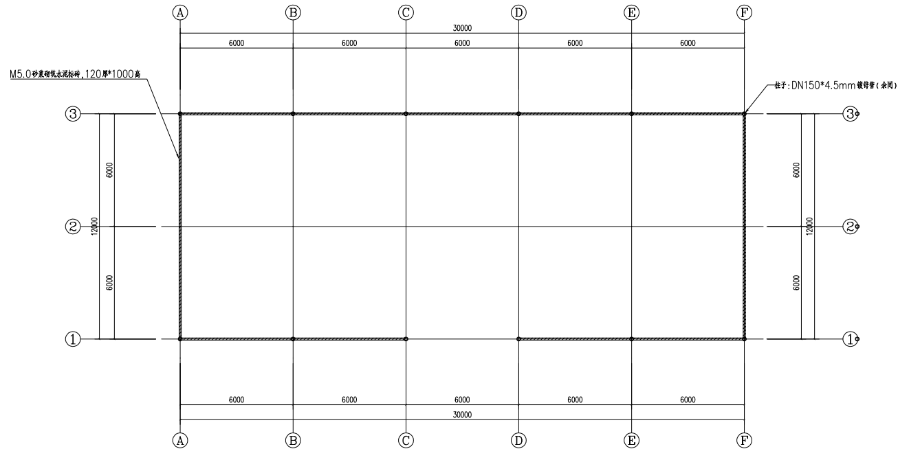
干湿分离区柱子平面布置图 1:100
