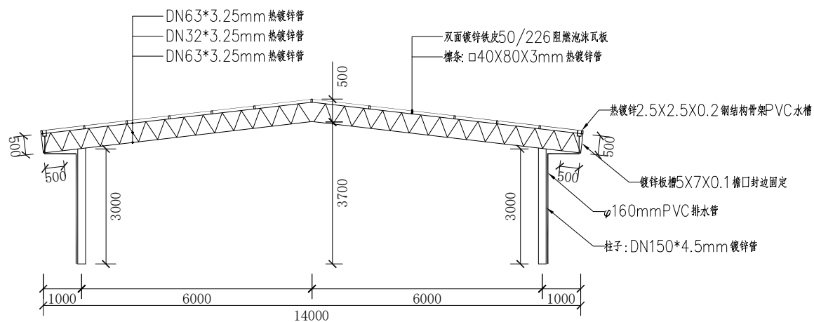
干湿分离区主樑处断面图 1:50
