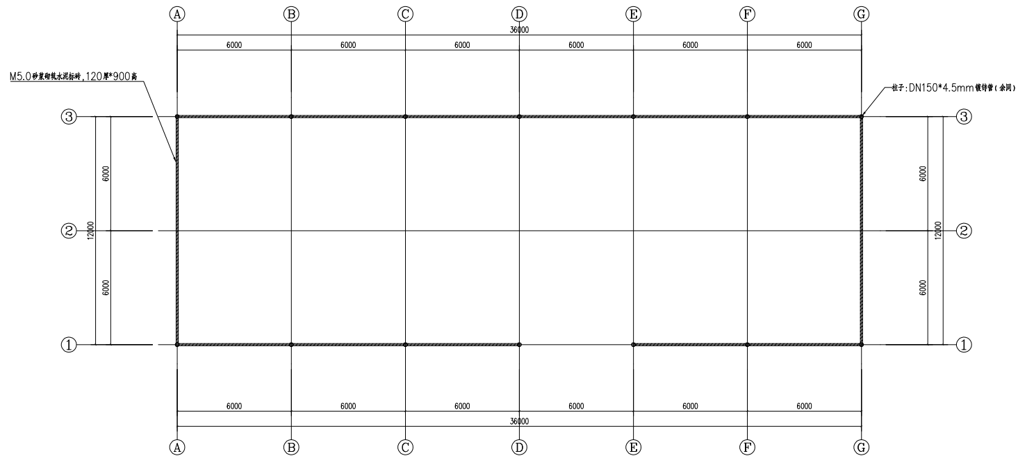
鵝棚(三)柱子平面布置图 1:100
