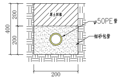
棚外饮水管安装断面图
