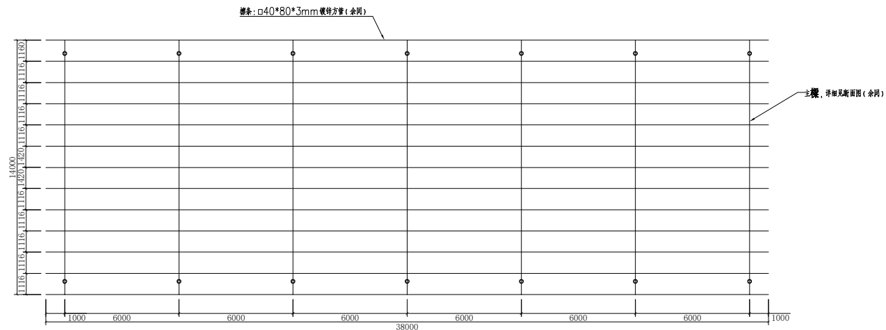
鹅棚(三)屋面檩条平面图 1:100
