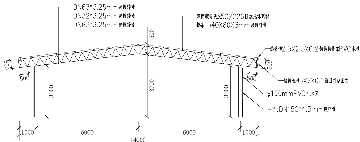
鵝棚(三)主樑處斷面圖 1:50
