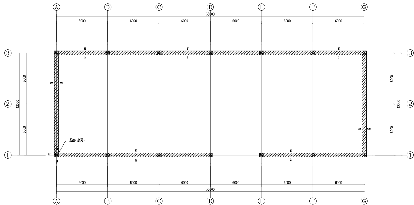
鹅棚(三)基础平面布置图 1:100
