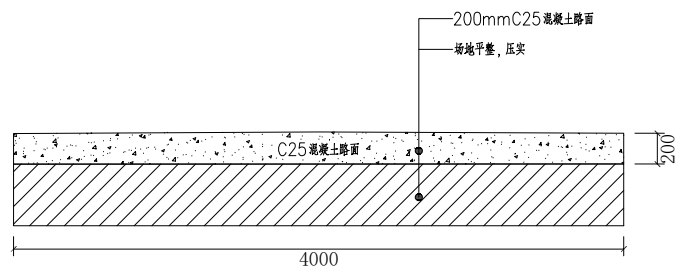
场内道路结构断面图 1:100
