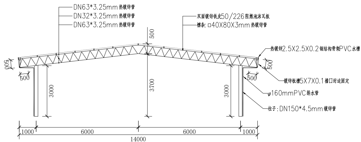
鵝棚(一)主樑處斷面圖 1:50
