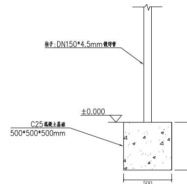
1-1剖面图
