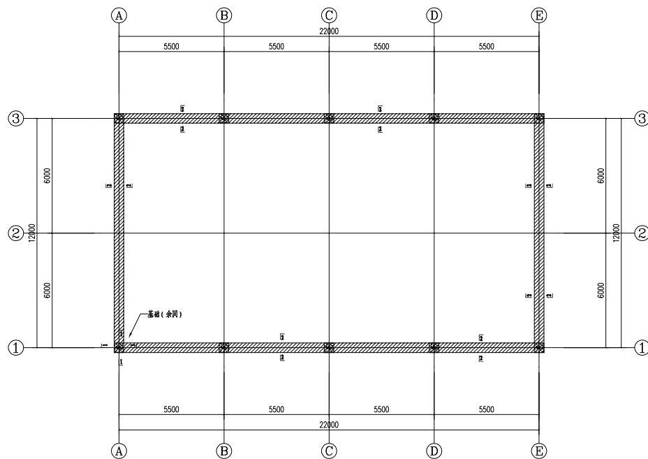
脱温棚基础平面布置图 1:100
