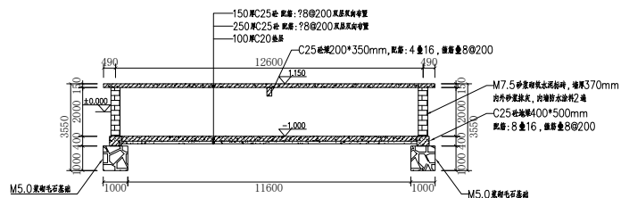
1-1剖面图 1:100
