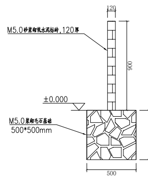
2-2剖面图
