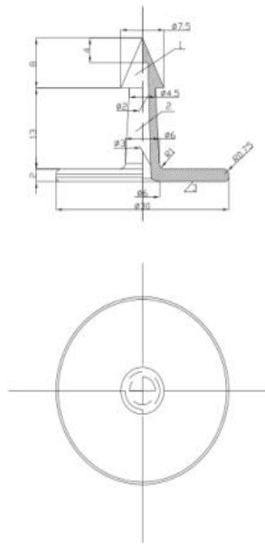
1-耳标头 2-耳标颈 3-耳标正面 牛耳标主标结构规格尺寸示意图(mm)
