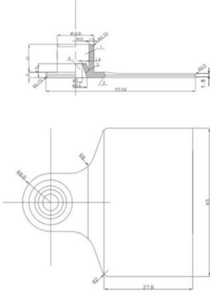
1-耳标锁扣 2-耳标副面 3-锁扣芯 4-锁孔 牛耳标辅标结构规格尺寸示意图(mm)
