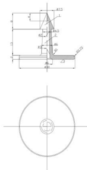
1-耳标头 2-耳标颈 3-耳标正面
