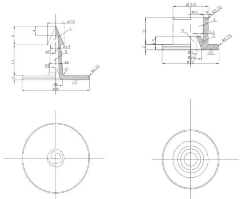
猪耳标主标、辅标结构规范尺寸
